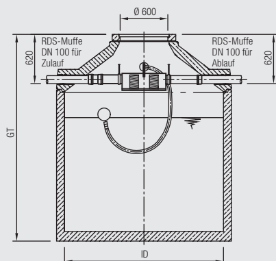
Schnitt Regenspeicher
