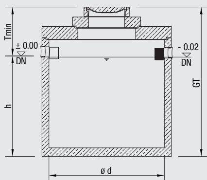
NeutraPit – Ausführung mit Abdeckplatte
