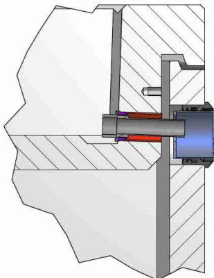
Detail Entwässerung 1:3,33
