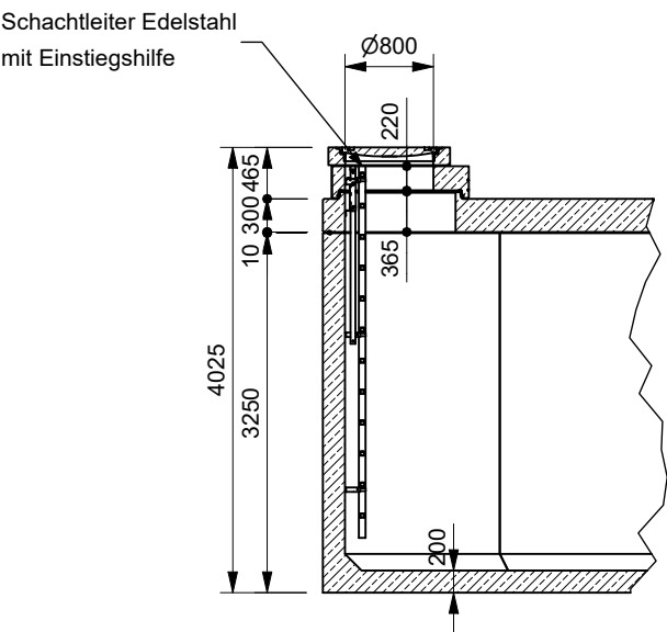
Schnitt B-B
