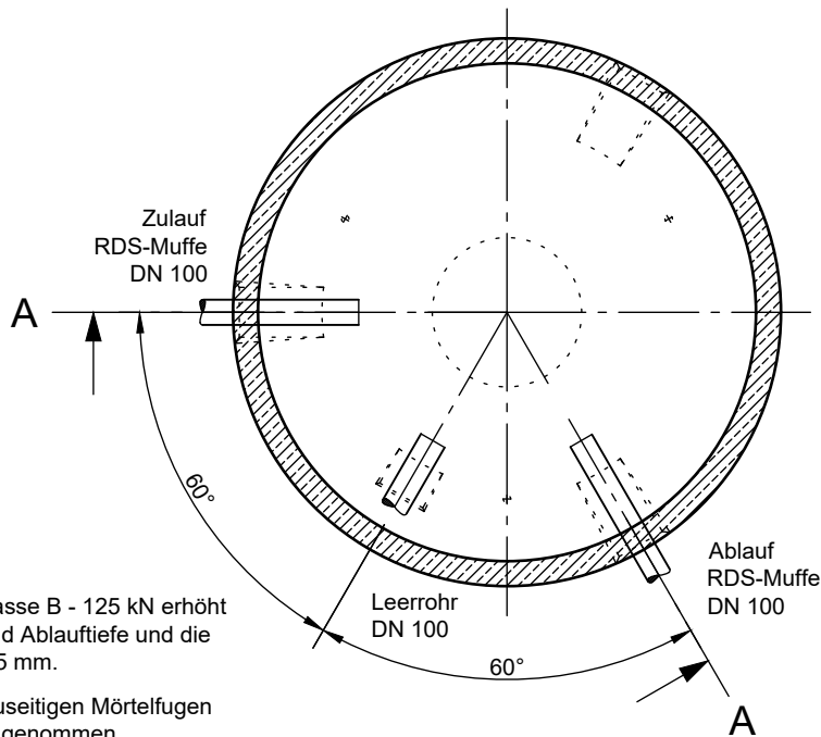
Grundriss
