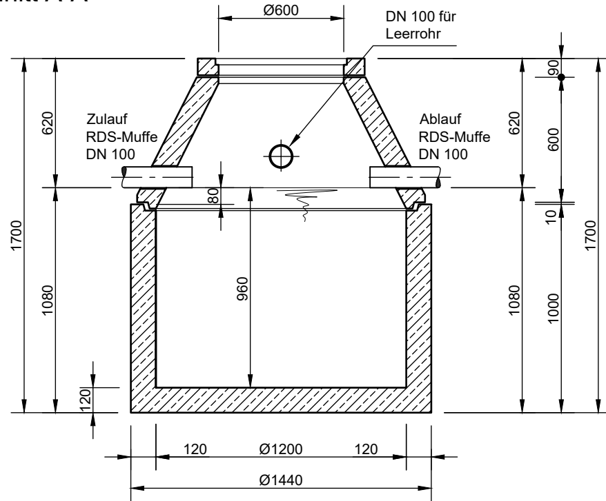
Schnitt A-A
