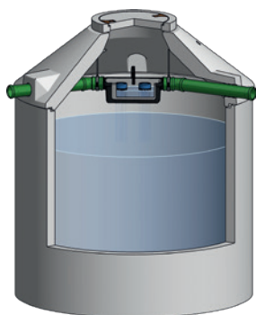
Zu- und Ablaufhöhe 620 mm unterhalb der Schachtabdeckung.
