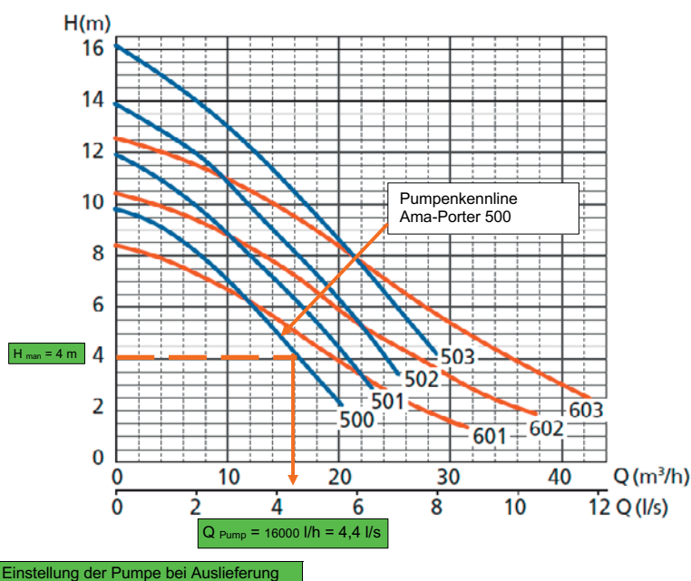
Kennlinien Ama-Porter 500 / 600
