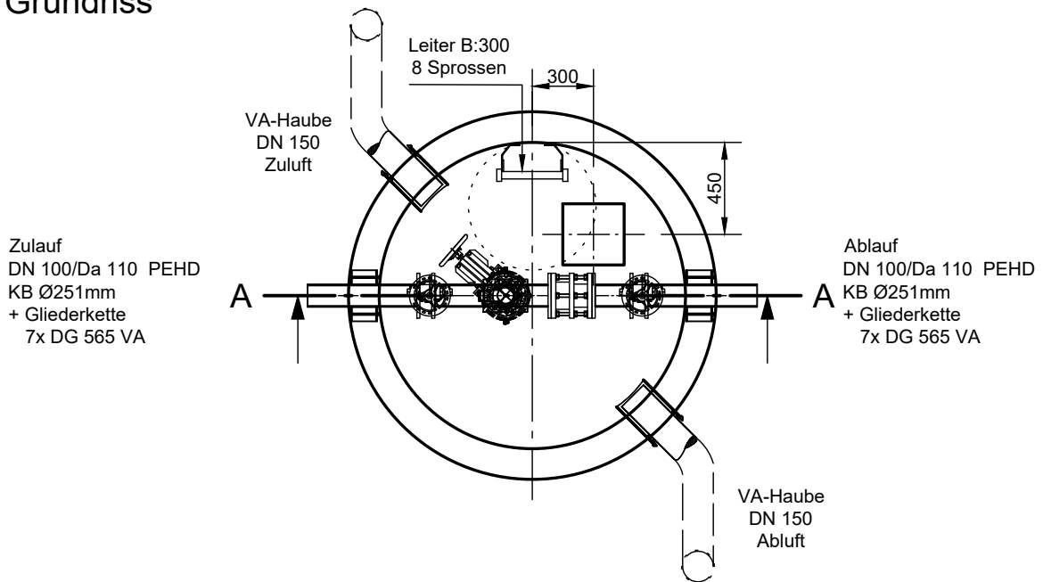
Grundriss
