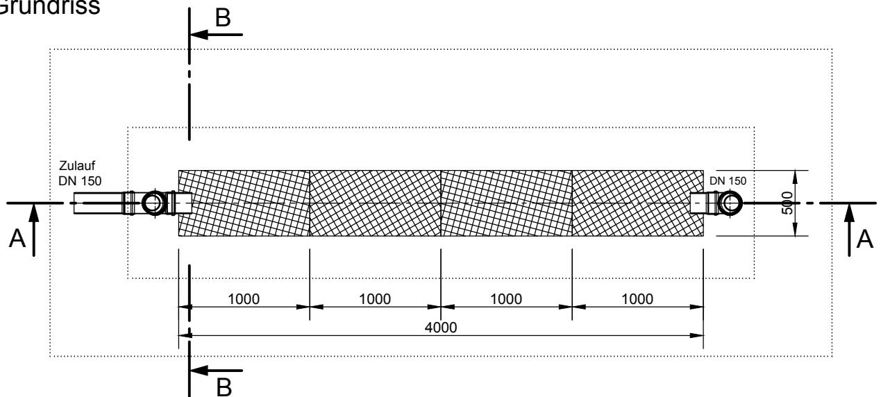
Grundriss
