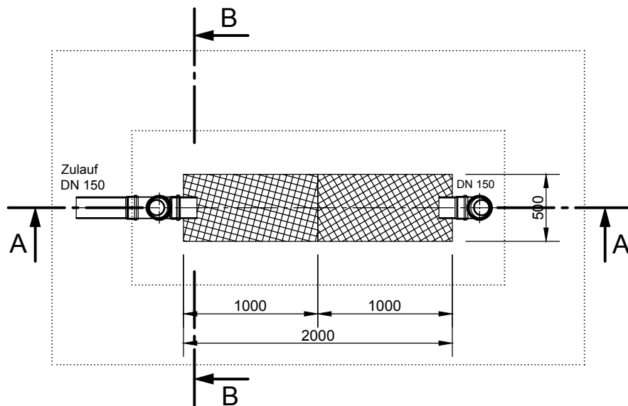
Grundriss
