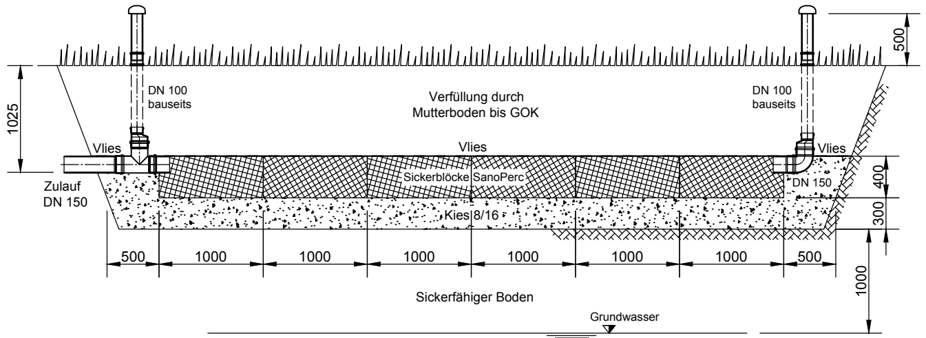
Schnitt A-A
