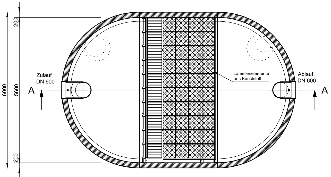
Grundriss
