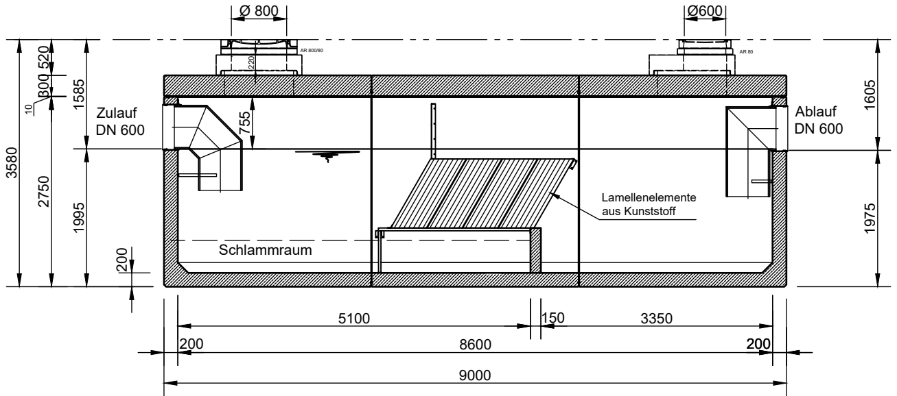
Schnitt A-A
