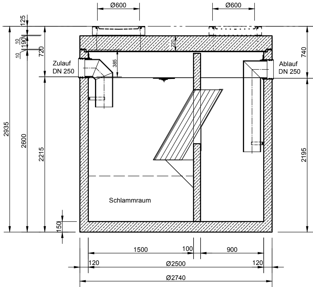
Schnitt A-A
