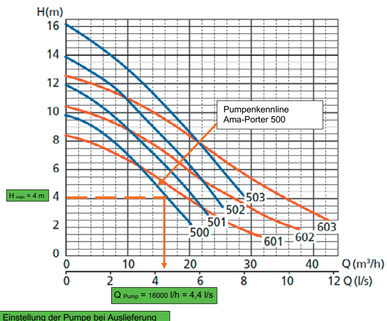
Kennlinien Ama-Porter 500 / 600
