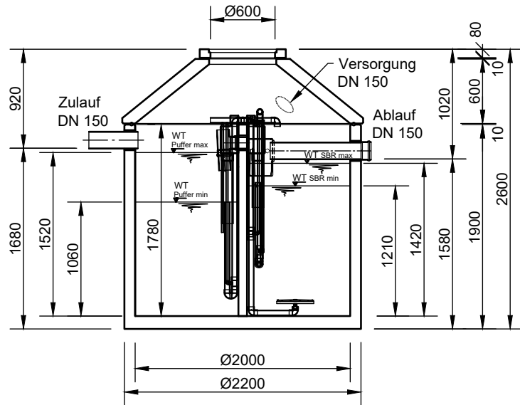
Schnitt A-A Schachtabdeckung Kl. A - 15, unbelüftet
