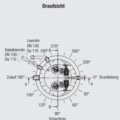
Draufsicht
