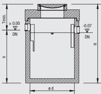
Ausführung mit Abdeckplatte und einer Öffnung bei Ø 1000 – Ø 1200
