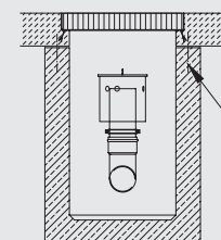
Variante 2 (Zarge bauseits in Ortbeton einbauen)
