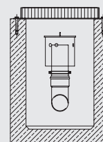
Variante 1 (Zarge gedübelt)
