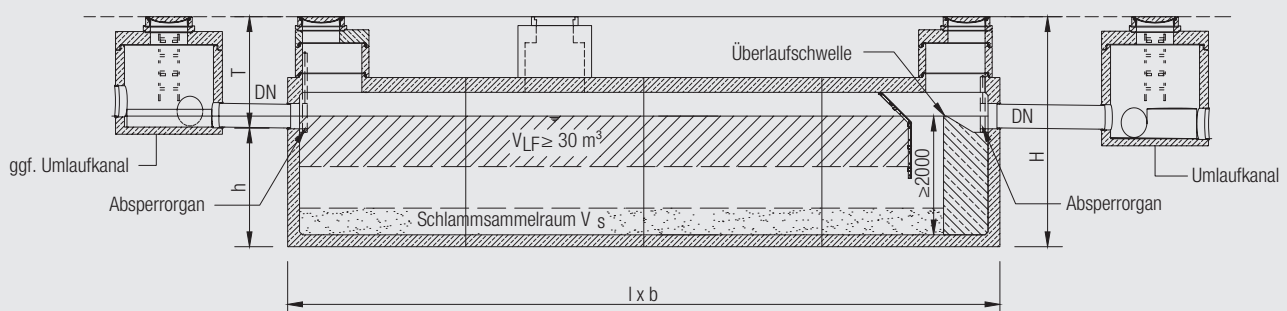
Schnitt
