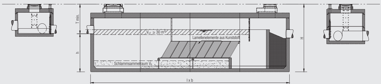
NeutraRiStWag mit Lamellenpaket (Ausführung REwSEW) – Schnitt
