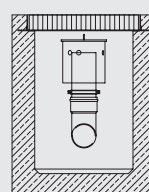
Standard (Zarge einbetoniert)
