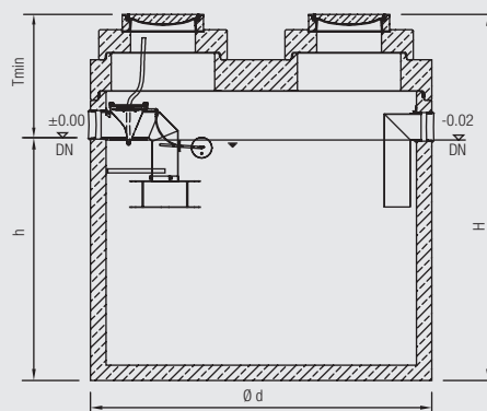
Ausführung ohne LF-Sammelbehälter
