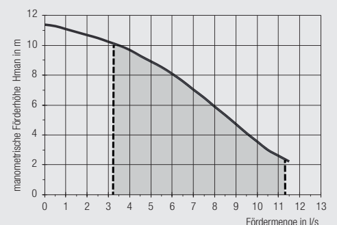
Pumpenkennlinie LevaPal
