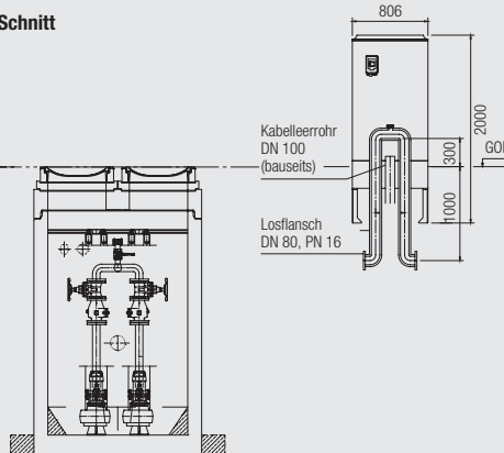
Schnitt
